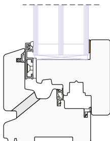
Nodo Inferiore finestra standard
