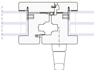
Nodo Centrale
