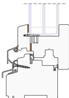
Nodo Inferiore
