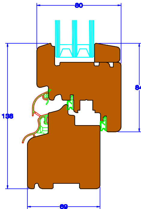
Nodo inferiore finestra
