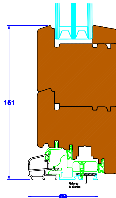
Nodo inferiore portafinestra
