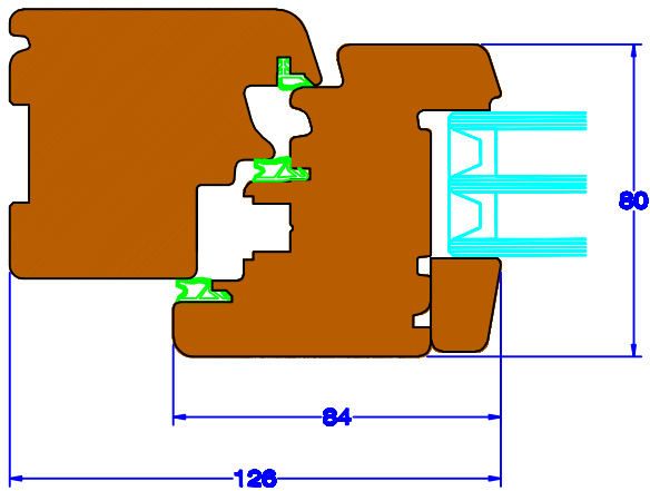
Nodo laterale e superiore
